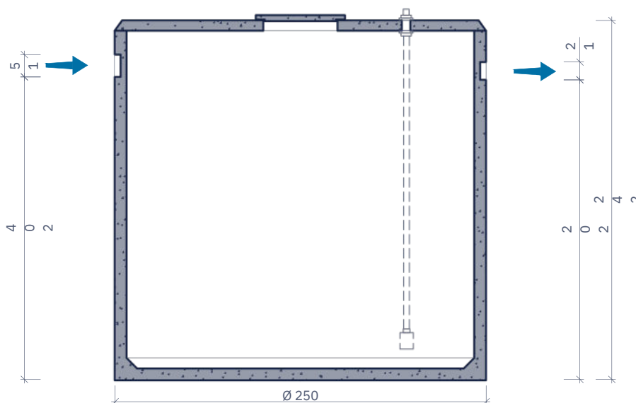
doorsnede coupe
